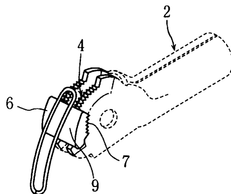
【使用状態を示す参考図 3】
